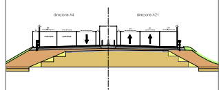
DA PK 4+870 A 7+400 SEZIONE TIPICA
